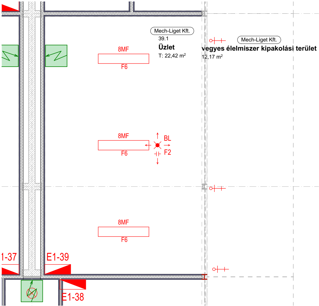
Bérői állmenyezeti terv
