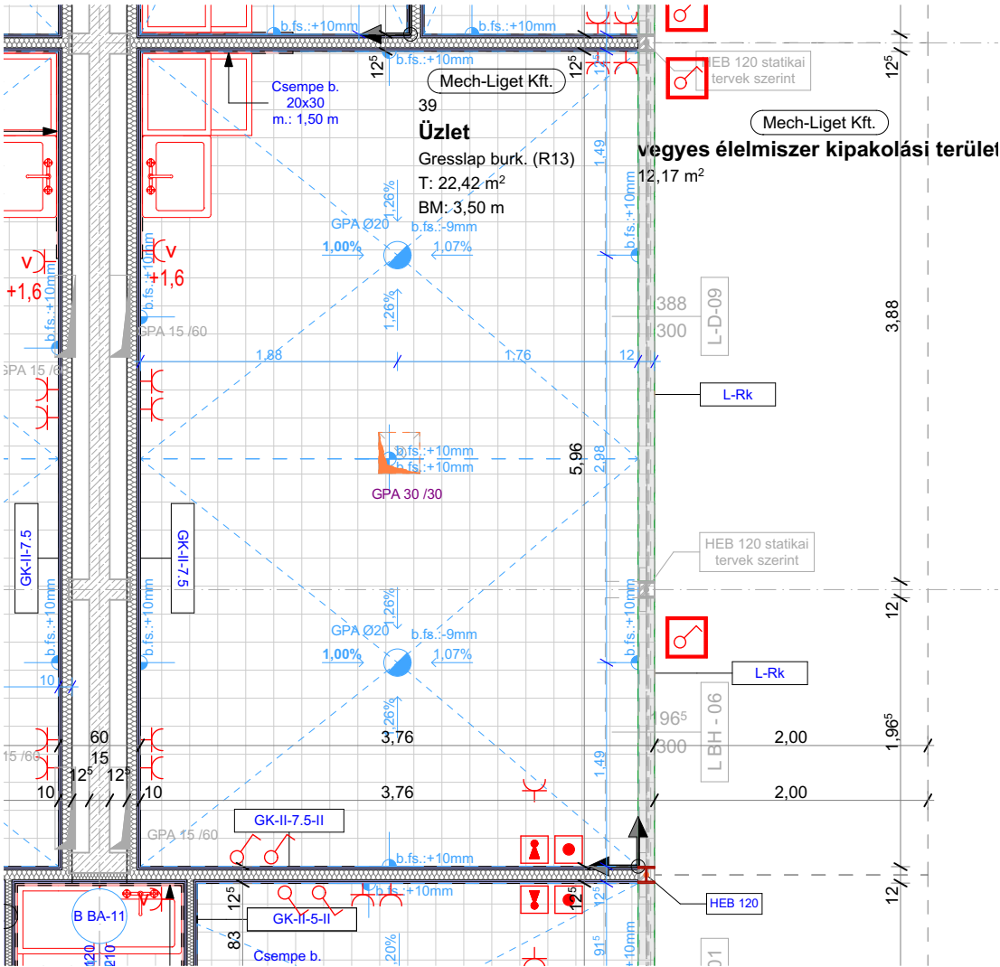
Bérői földszinti alaprajz
